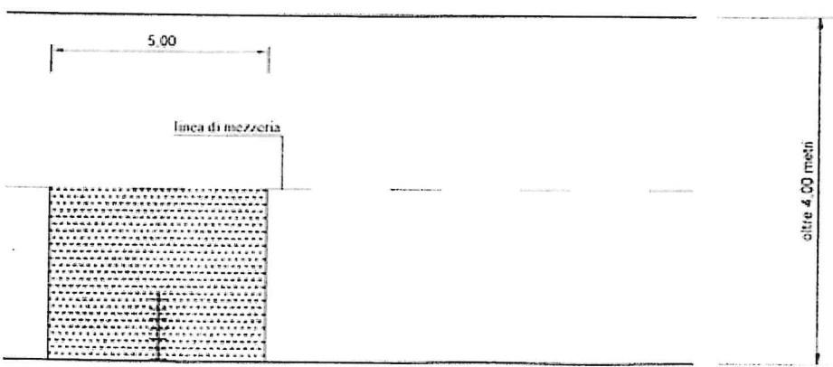
figura 8 scavo trasversale alla carreggiata
